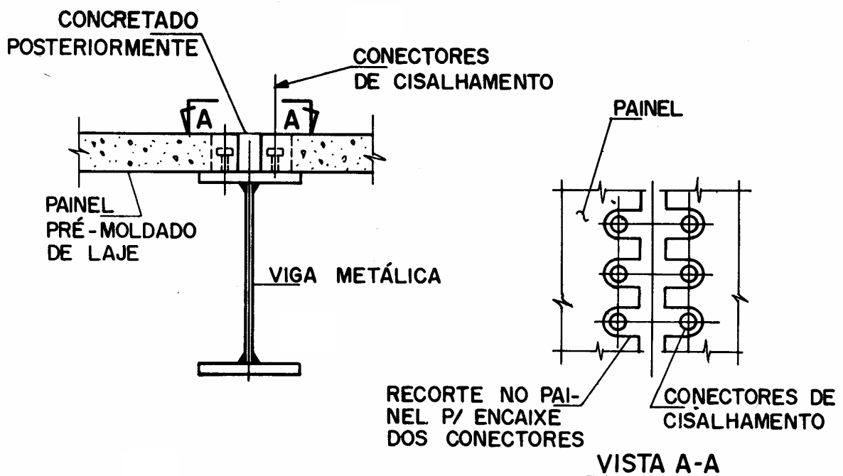
(C) LAJE PRÉ-MOLDADA
