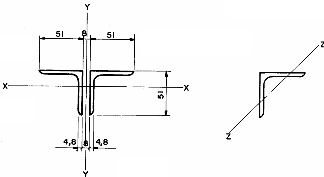
r_x = 1,58\text{cm} (RAIO DE GIRAÇÃO DA SEÇÃO EM RELAÇÃO AO EIXO X) r_y = 2,32\text{cm} (RAIO DE GIRAÇÃO DA SEÇÃO EM RELAÇÃO AO EIXO Y) r_z = 1,00\text{cm} (RAIO MÍNIMO DE GIRAÇÃO DE UMA CANTONEIRA ISOLADA) Fig. 30 – Seção da Diagonal
