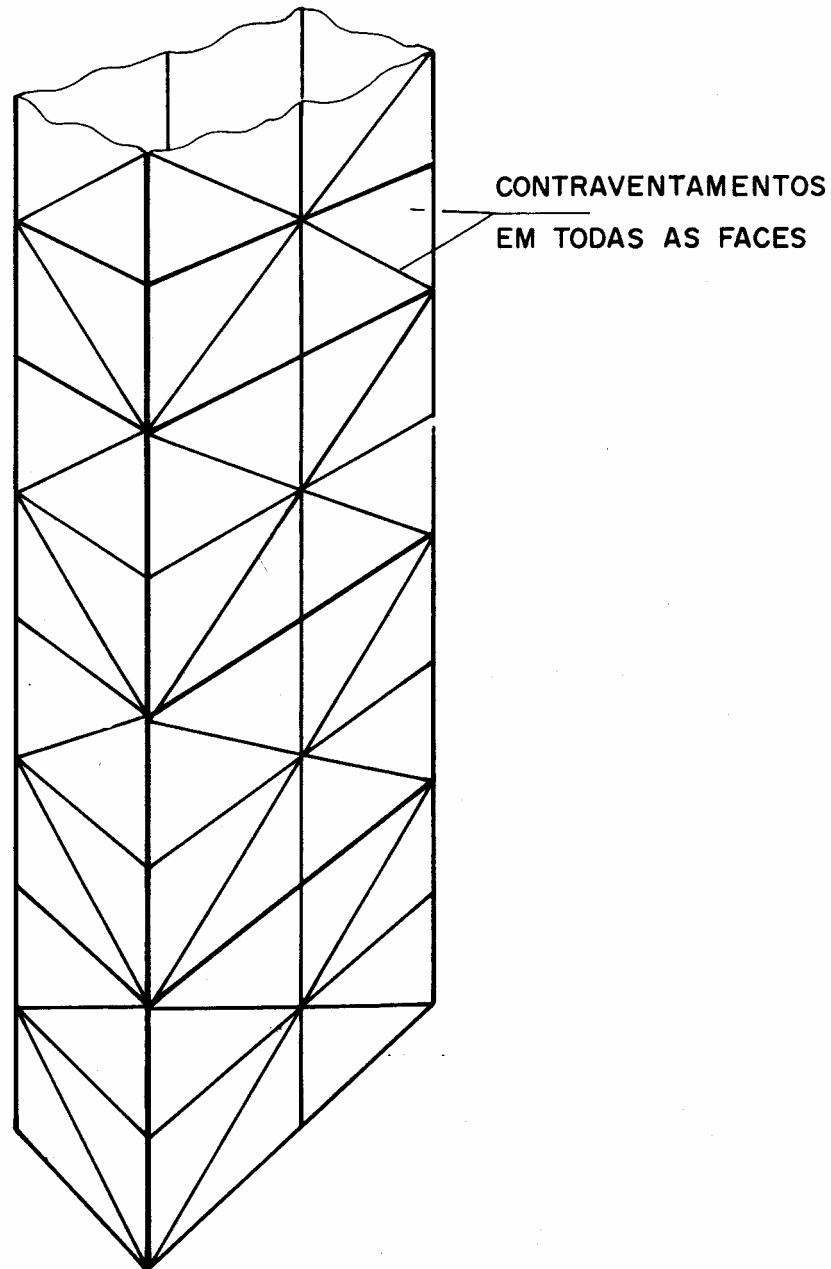
Fig. 7 – Estrutura Tubular
