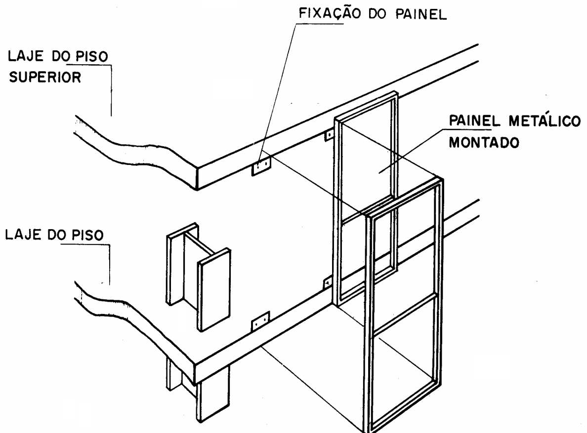
Fig. 14 – Parede Externa com Painel Metálico
