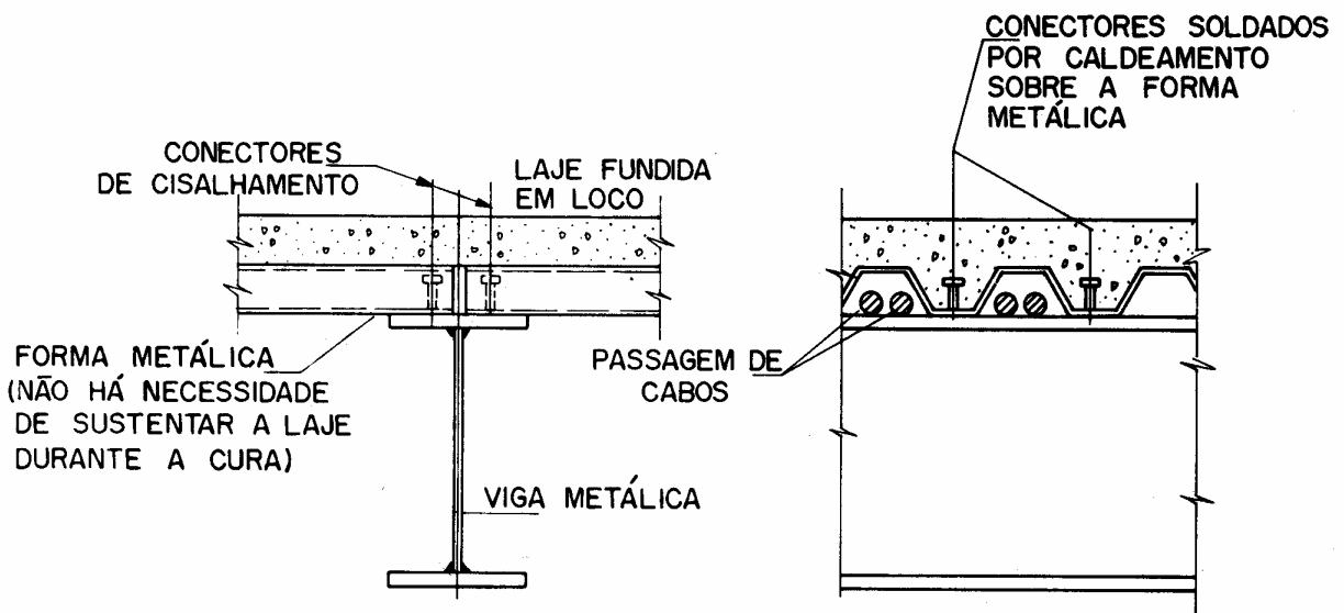
(B) LAJE COM FORMA METÁLICA
