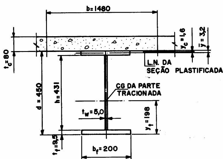
VIGA MISTA
