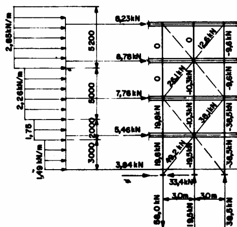
Fig. 28 – Esforço no Contraventamento
